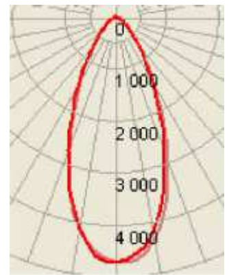
● 配光曲線
